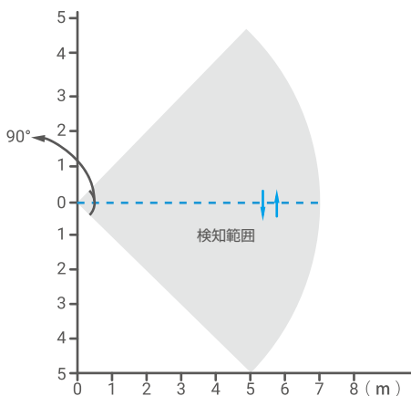
図 2 検知範囲を上から見た図
