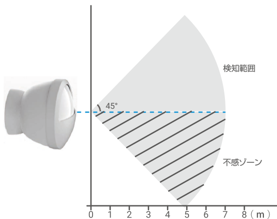
図 2 検知範囲を上から見た図
