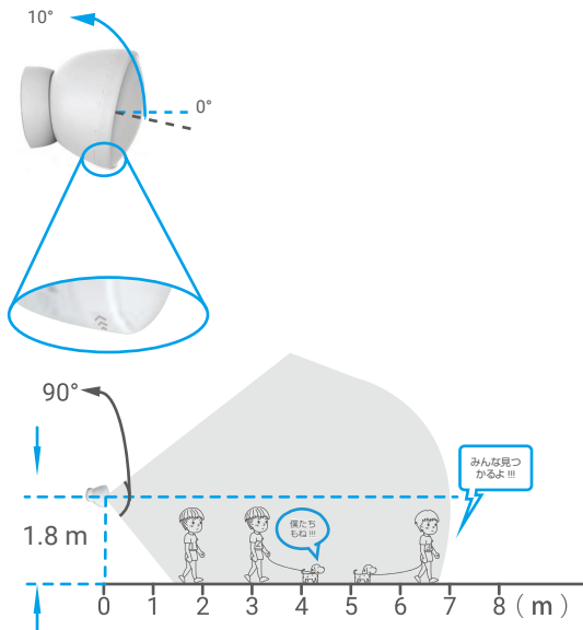
図 1 検知範囲を横から見た図
